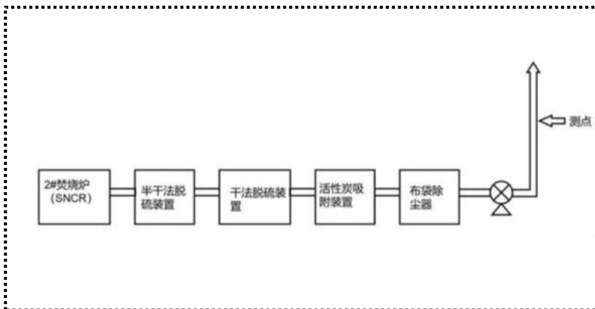
测点示意图
