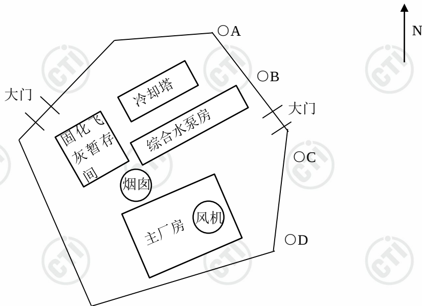
附：工业废气（无组织）测点示意图
