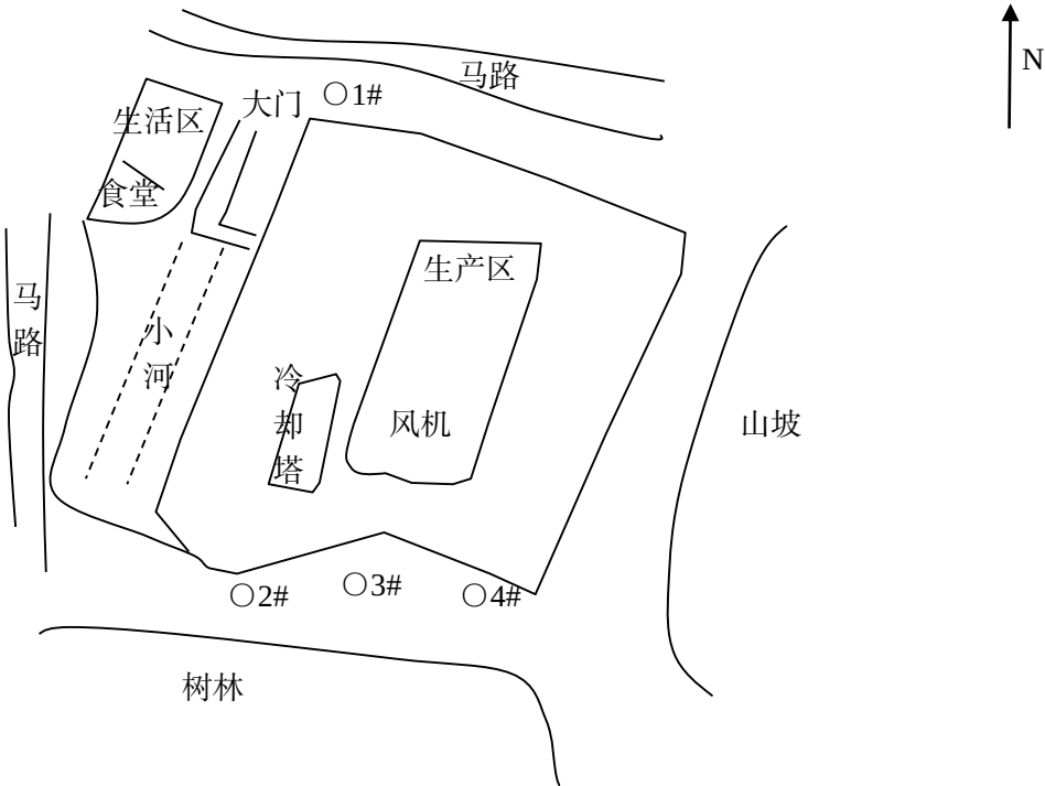
附：工业废气（无组织）测点示意图
