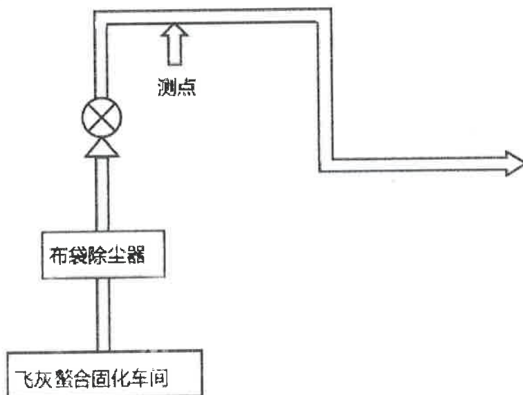
测点示意图
